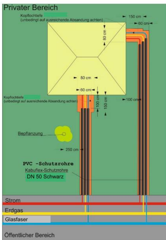
Abbildung 1 – Zulässige Verlegung
